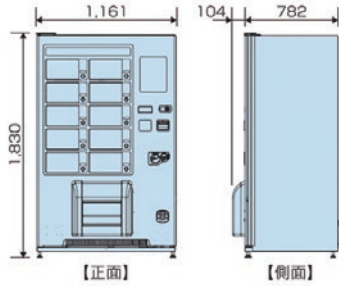
●外形図 (単位:mm)
